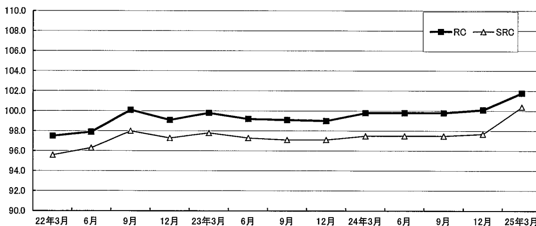
建築費指数
