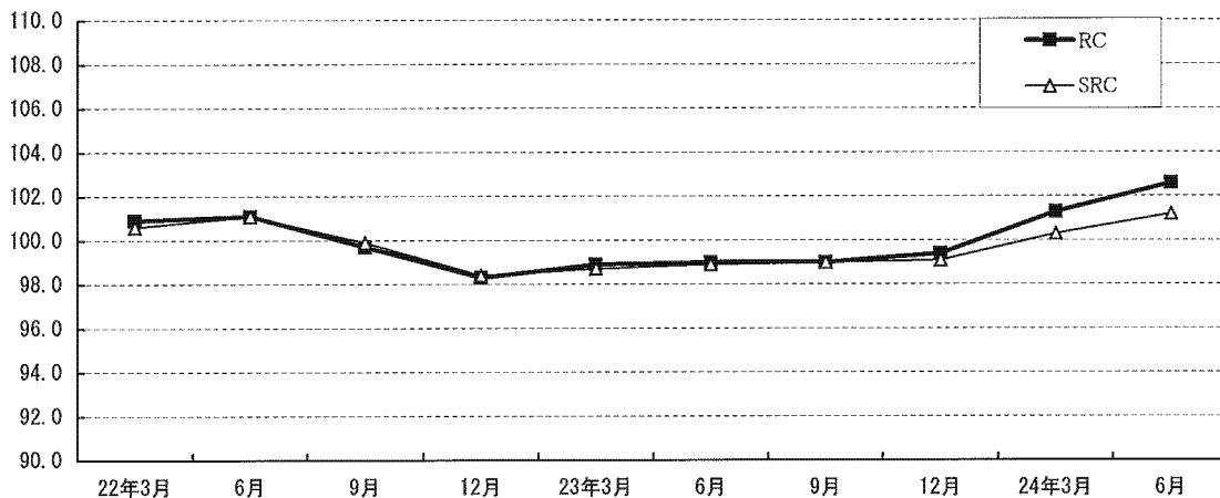
建築費指数
